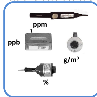
D13.000.0 Gaskonzentrations-Sensoren
